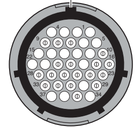
Receptacle Socket
